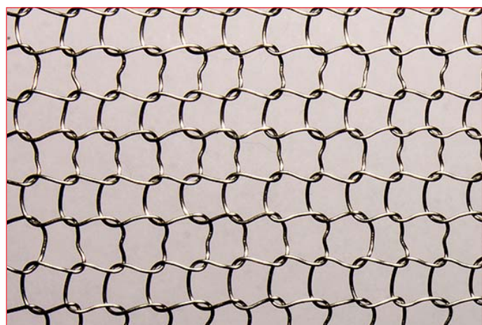
Photographie agrandie du grillage en mailles standard de KnitMesh. La finition est en acier inoxydable 304 tricoté. D'autres finitions sont disponibles sur demande
