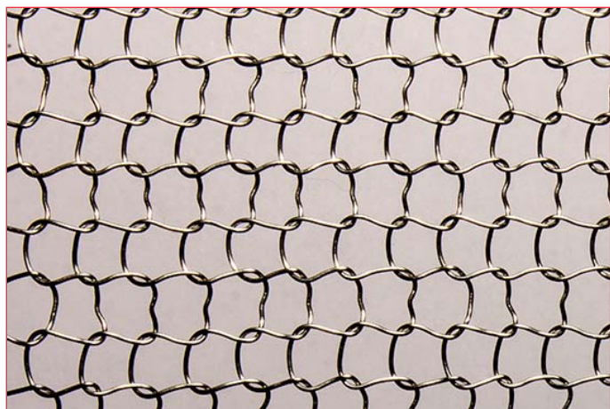
Fotografía aumentada de la malla de cerramiento 'estándar' de KnitMesh. Acabado en acero inoxidable 304. Otros acabados disponibles previa solicitud
